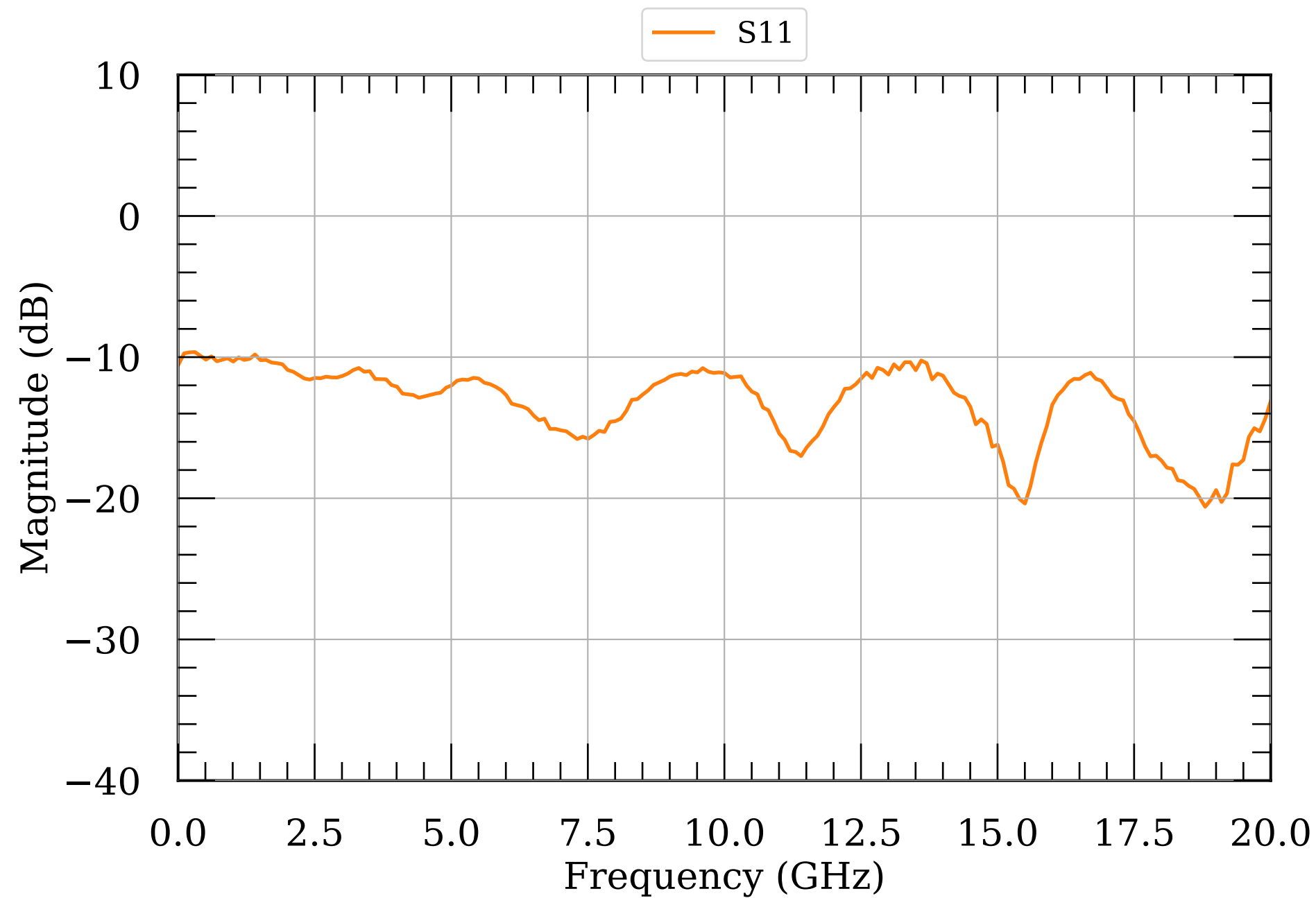
LNA S-params module073
